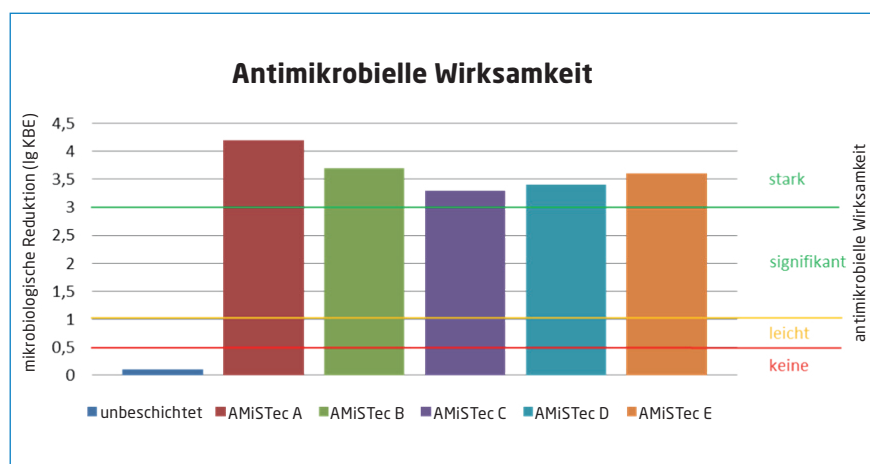
Abbildung 6: Antimikrobielle Wirksamkeit der AMiSTec-Prüfkörper nach JIS Z 2801. (N=3)
